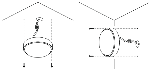
Рис. 2. Пример монтажа
